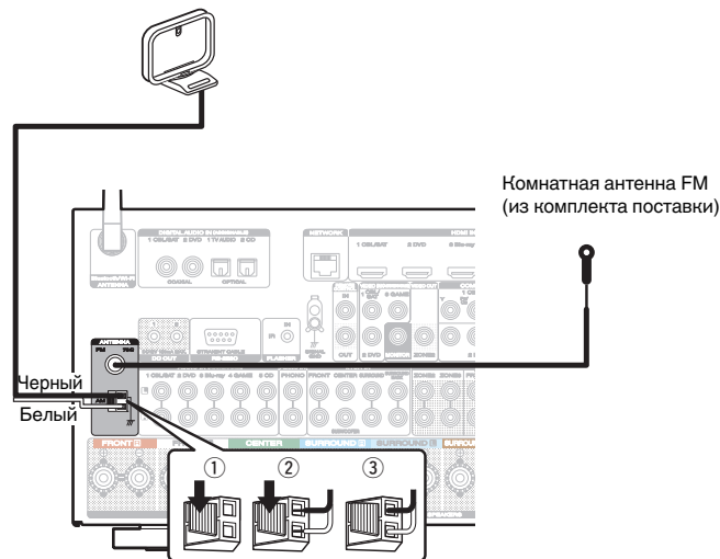
Рамочная AM-антенна (из комплекта поставки)
